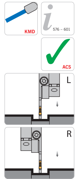
Rechter Halter und linkes Modul montiert Halter höhenstellbar Rechtes Modul alternativ Right holder and left module shown Height adjustable holder Right module alternative Adattatore destro e modulo sinistro in figura Adattatore registrabile in altezza Modulo destro alternativa
