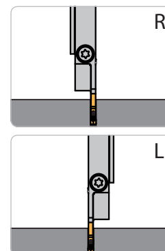
Linker Halter und linkes Modul montiert Left holder and left module shown Adattatore sinistra e modulo sinistra in figura
